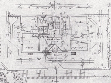
FÖLDSZINTI ALAPRAJZ M 1:100 ISMÉTELTEN MÓDOSÍTOTT
