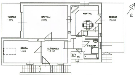
FÖLDSZINTI ALAPRAJZ netto 75 m 2
