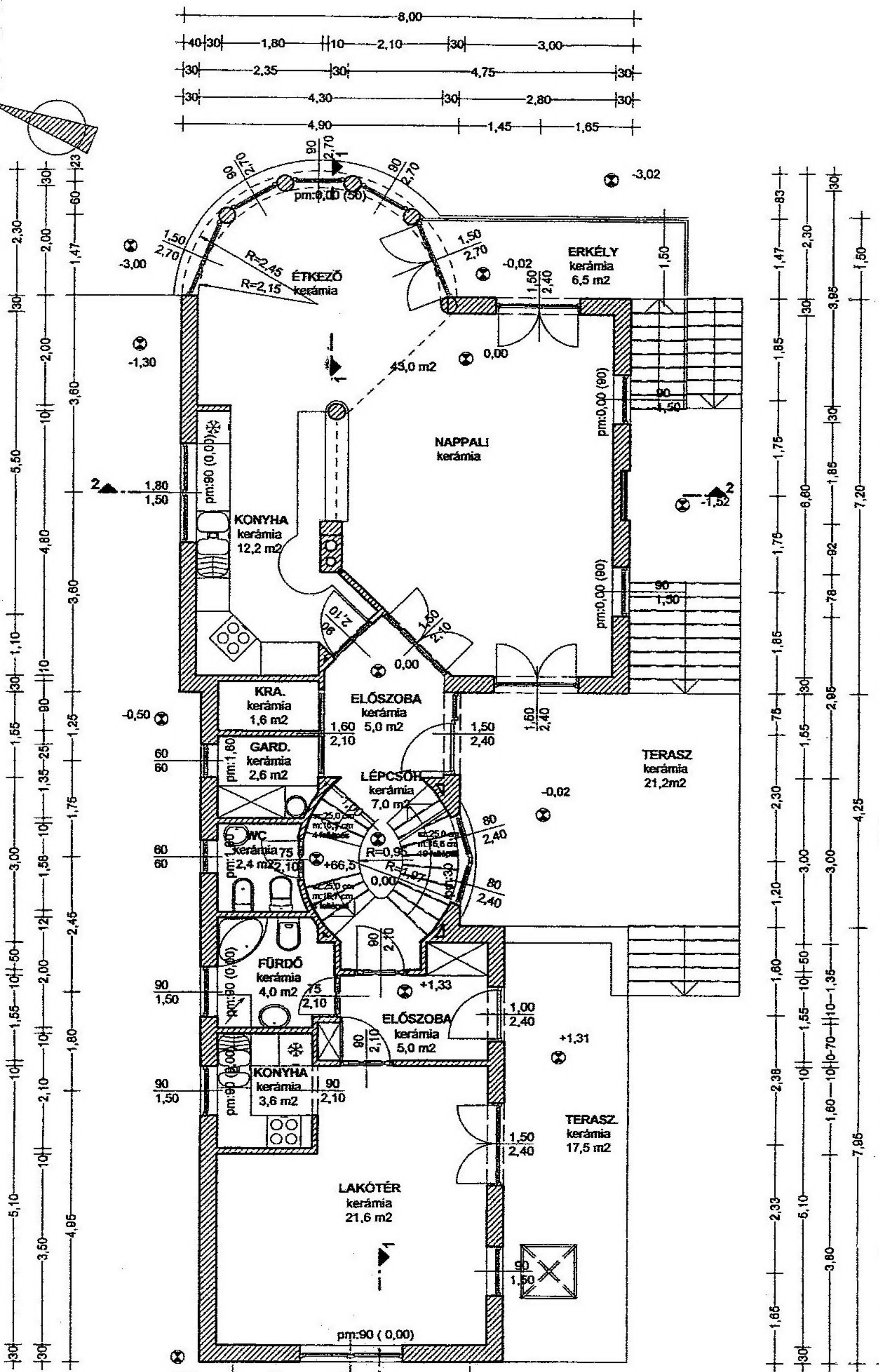
FÖLDSZINTI ALAPRAJZ M 1:100
